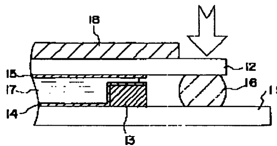
11, 12 基板 13 液晶止め用凸部 14, 15 垂直配向膜 16 シール材
